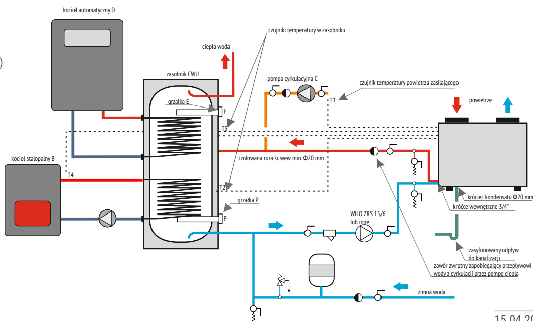
Kocioł stałopalny podłączyć jak w schemacie nr 5.
